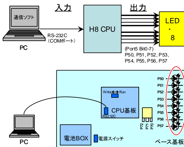
図 15.1 この実験の入出力構成と、配線図
