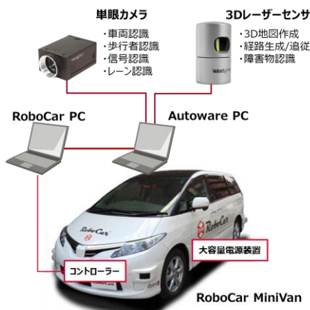
<Autoware システム構成例>
